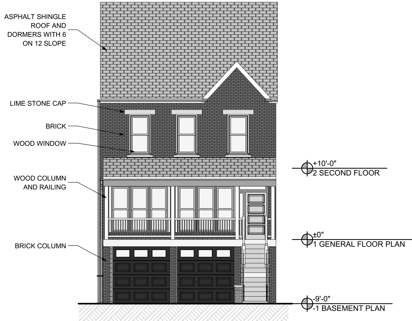
1 FRONT ELEVATION SCALE: 1/8" = 1'-0"
